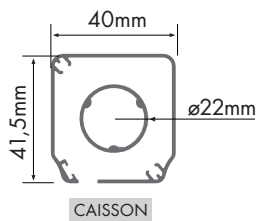
CAISSON
