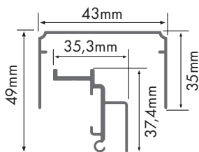
COULISSE SUPÉRIEURE
